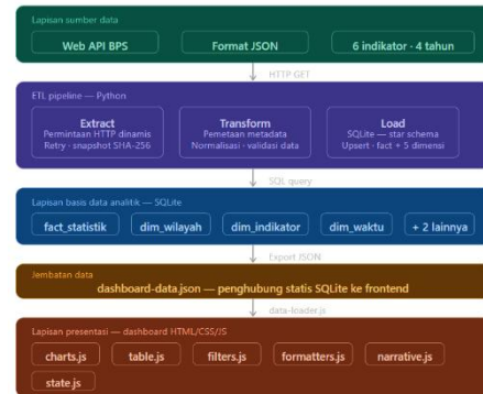
Gambar III.2 Arsitektur Sistem
